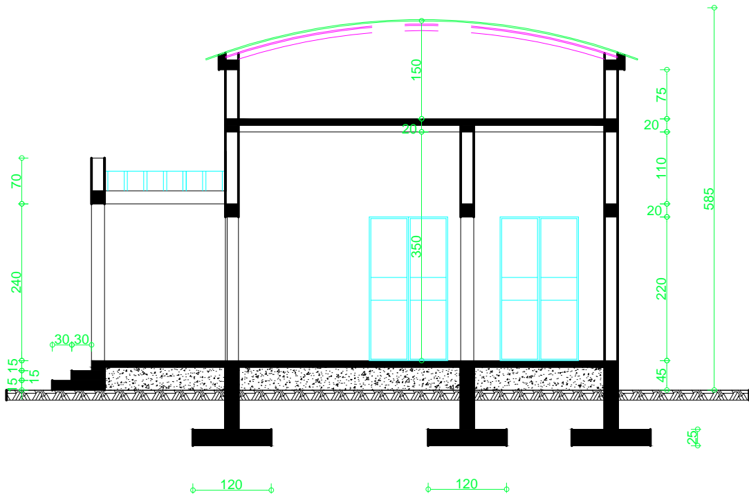
COUPE A-A
